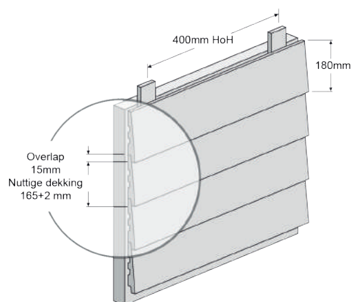
22 x 180 Bevel
