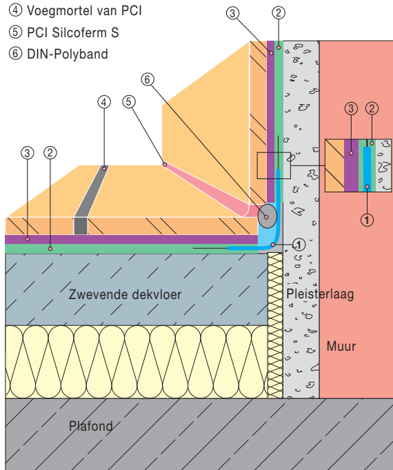
Detail: Aansluiting vloer/wand
