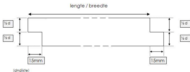
Fig. 1 – sponning
